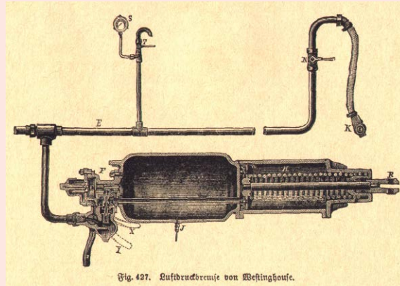
Eisenbahnluftdruckbremse. (Hrsg. H. Samter [1901]: Das Reich der Erfindungen [Jubiläumsausgabe ed.], Berlin und Leipzig: Verlag von W. Herlet/Wikimedia CC)
